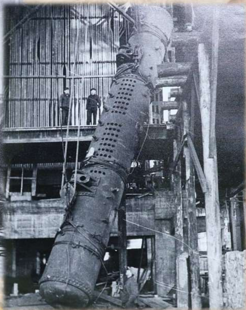
Монтаж котлоагрегата № 2 НГА Ф.Р-75.Оп.1.Д.2541
