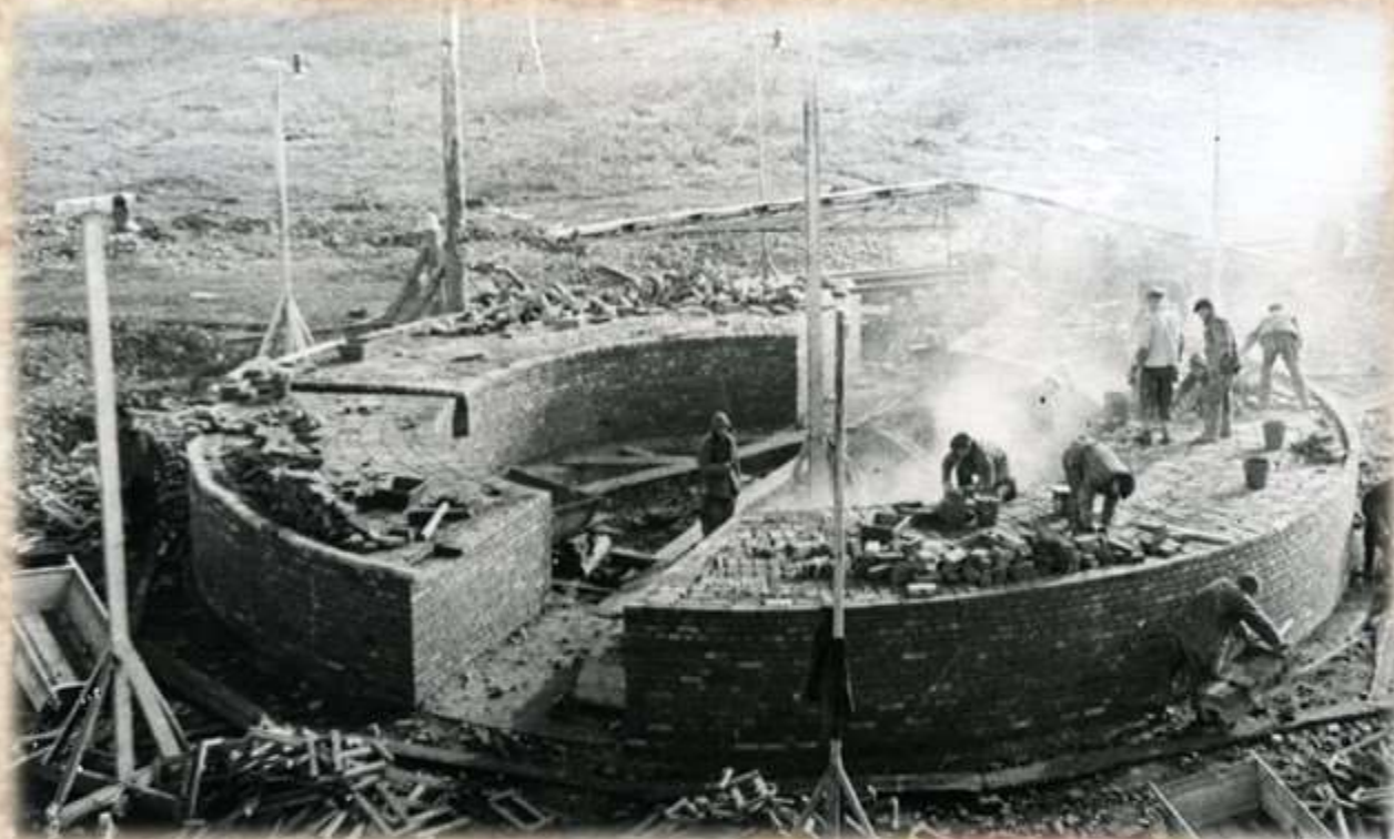
Строительство Большого металлургического завода. Кладка цоколя под трубу 140 м. НГА Ф.Р-75.Оп.1.Д.1786
