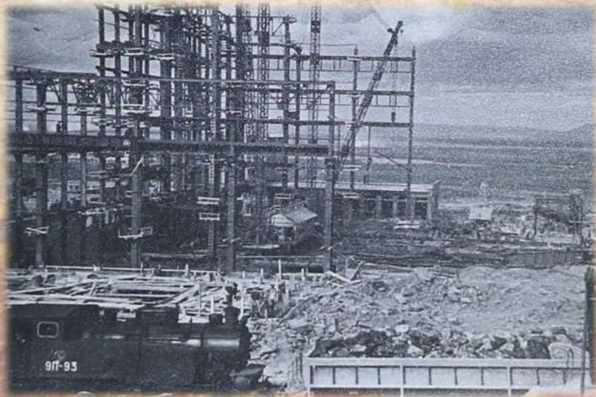
Строительная площадка ТЭЦ-1. Возведение здания НГА Ф.Р-75.Оп.1.Д.2530
