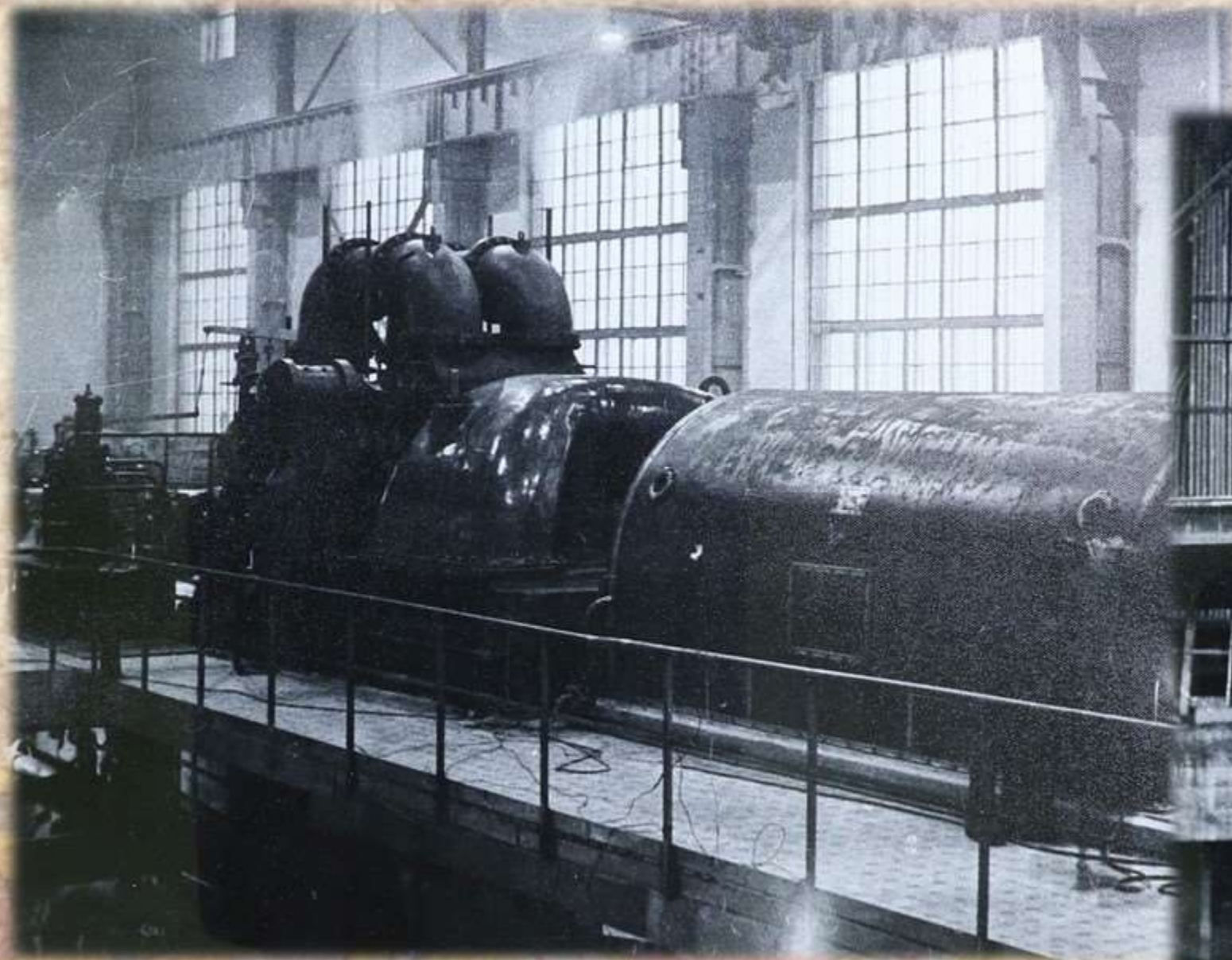
Турбинный цех ТЭЦ-1. НГА Ф.Р-75.Оп.1.Д.2538
