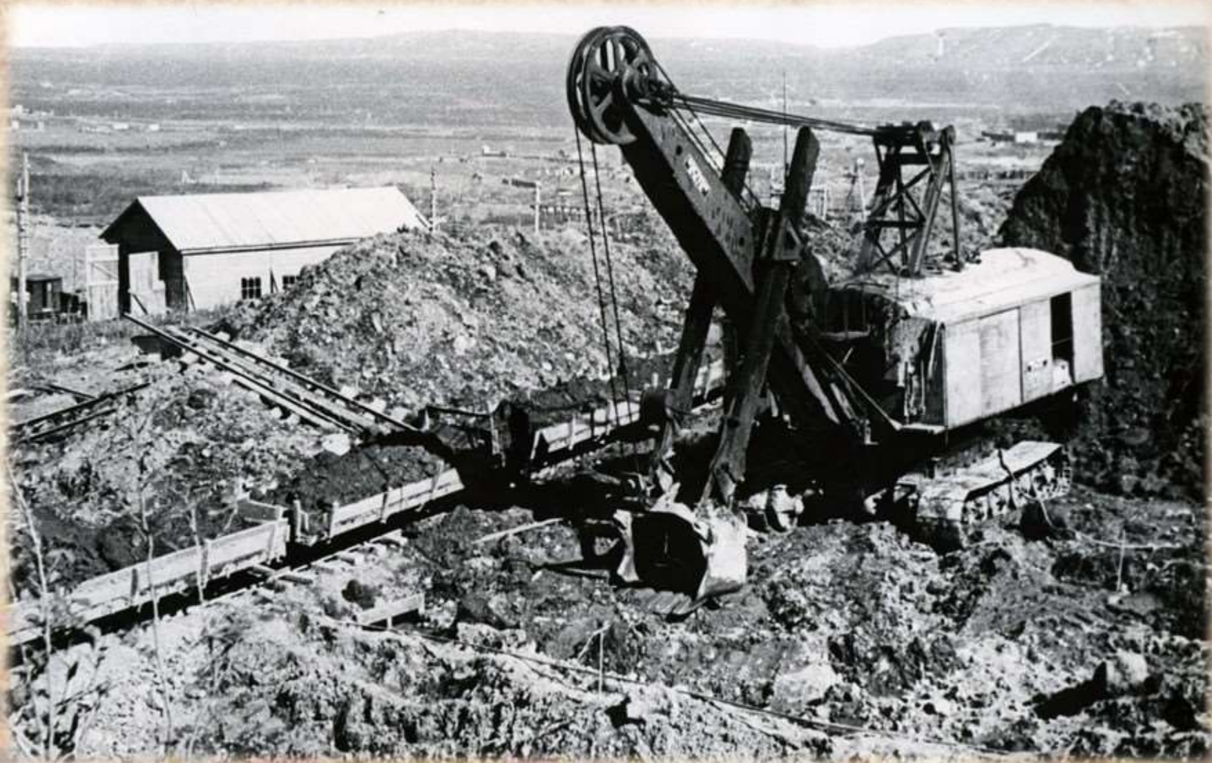
Земляные работы на строительстве БОФ. 1944 г. НГА Ф.Р-75.Оп.1.Д.1941
